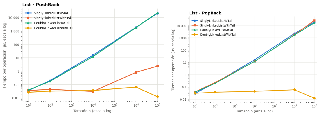
Figura 1. PushBack (izq.) y PopBack (der.) en las 4 listas.
