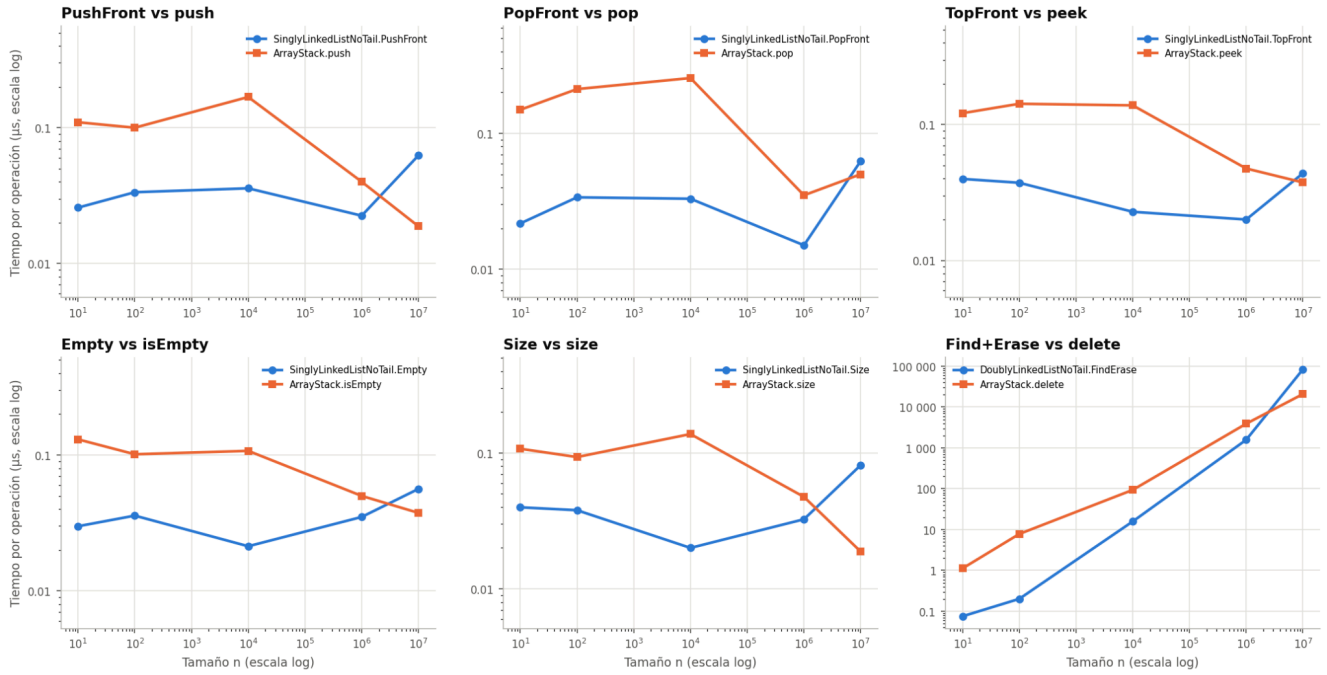
Figura 8. List (simple sin cola; doble sin cola para Find+Erase) vs. ArrayStack.
