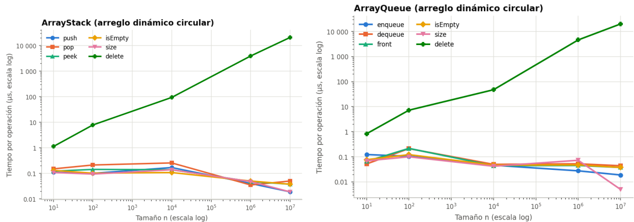
Figura 6. Métodos de ArrayStack (izq.) y ArrayQueue (der.).
